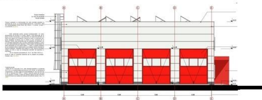
Figura 6 Noua clădire propusă
